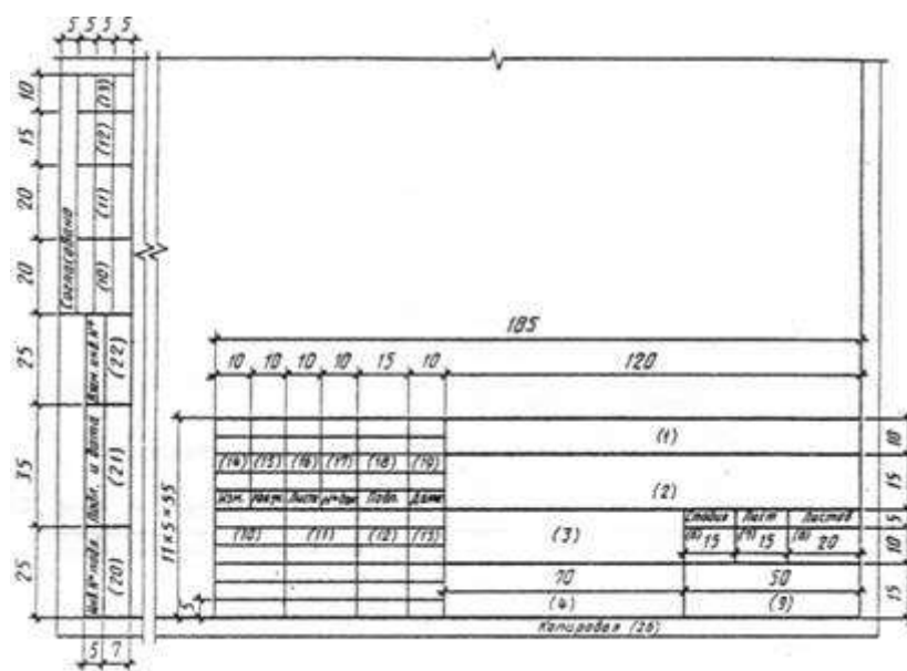
Форма 4 - Для чертежей строительных изделий (первый лист)
