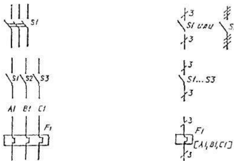
а - многолинейное изображение; б - однолинейное изображение.
